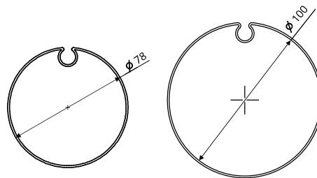
ROLLER TUBE | RURA NAWOJOWA BARRE D'ENROULEMENT | TUCHWELLE
