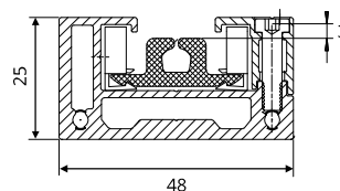
GS 25 SIDE GUIDE WITH STANDARD ZIP INSERT ROWADNICA GS 25 ZE STANDARDOWĄ WKŁADKĄ ZIP GUIDE GS 25 AVEC INSERT ZIP STANDARD FÜHRUNGSSCHIENE GS 25 MIT STANDARD-ZIP-EINLAGE
