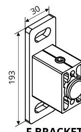
F BRACKET UCHWYT PROWADNICY F SUPPORT DE GUIDE F FASSADENHALTERUNG
