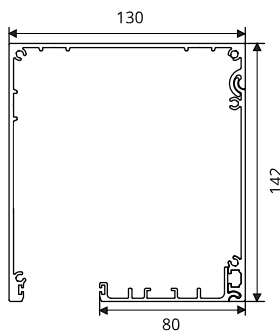
CASSETTE 130 | KASETA 130 CAISSON 130 | KASSETTE 130
