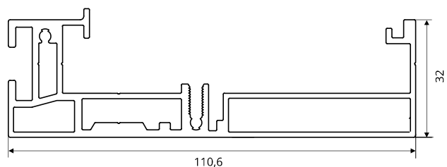
GUIDE | PROWADNICA GUIDE | FÜHRUNGSSCHIENE
